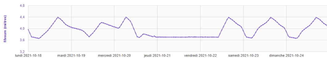
📡 Niveau : SUR_LANGENNERIE - MES_NIV_BACHE_800m3 (mètres)
